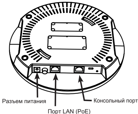
Рисунок 2. Задняя панель DWL-6610AP
