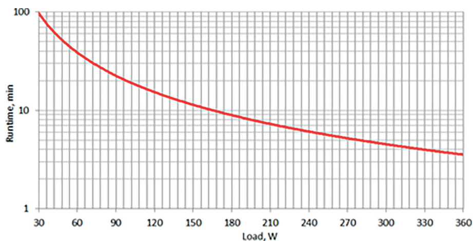
Figura 4. Grafico della durata della batteria di INFOPDU600 / INFOPDU600PL / INFOPDU600LCD
