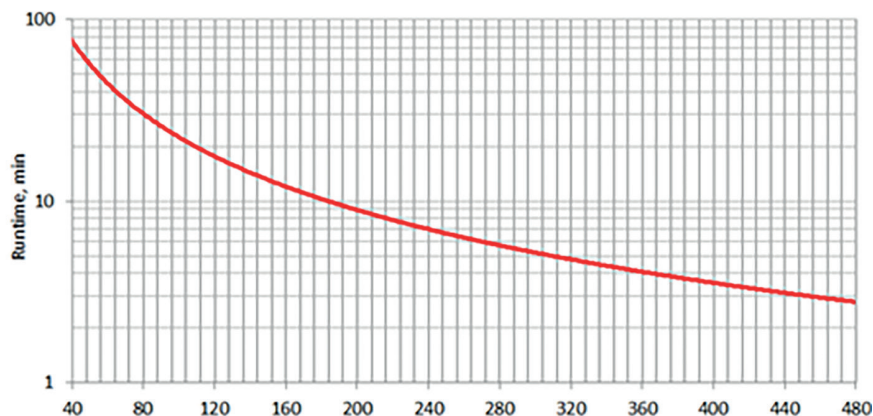
Figura 5. Grafico della durata della batteria di INFOPDU800 / INFOPDU800PL / INFOPDU800LCD
