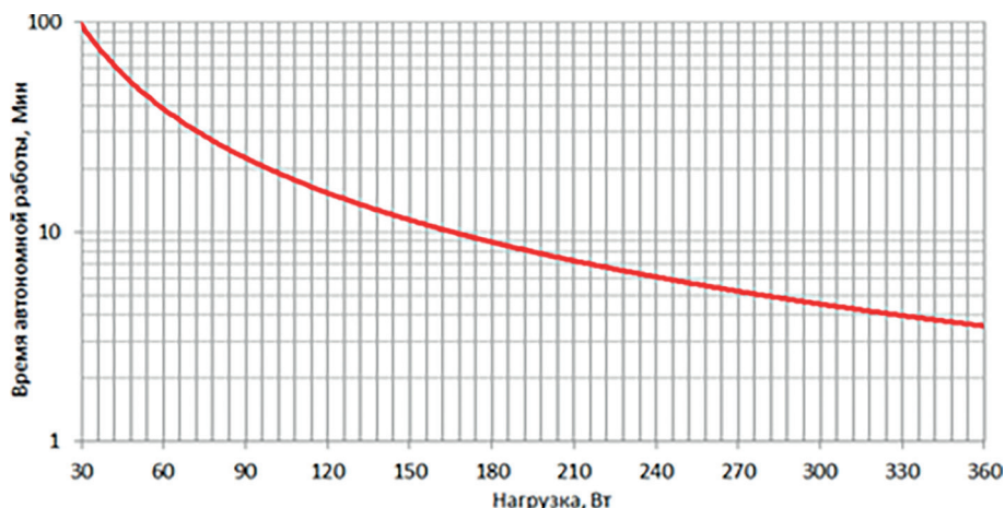
Рисунок 4. График автономной работы INFOPDU600 / INFOPDU600PL / INFOPDU600LCD
