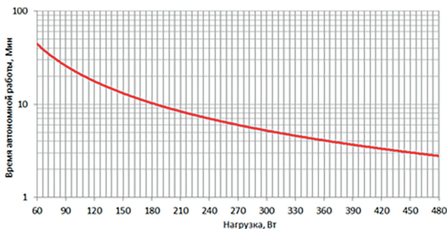
Рисунок 5. График автономной работы INFOPDU800 / INFOPDU800PL / INFOPDU800LCD
