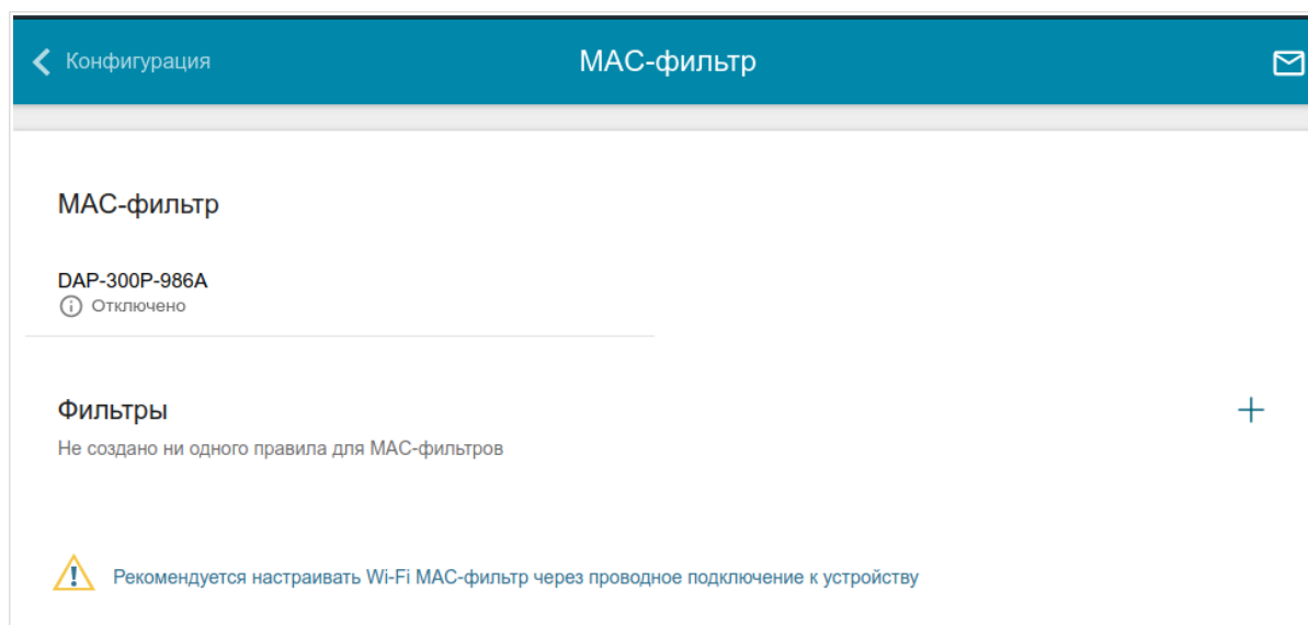
Рисунок 94. Страница для настройки MAC-фильтра для беспроводной сети.
